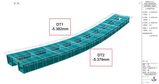
LC-2 하중 재하시 처짐형상
