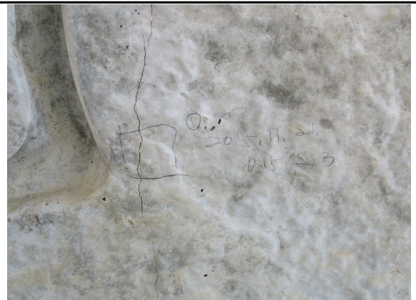
교대 A1 전면 균열 발생(점검일:2015.12)
