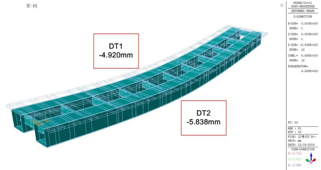
LC-3 하중 재하시 처짐형상
