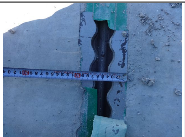
신축이음 A2 유간 측정
