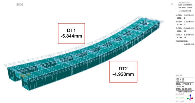
LC-1 하중 재하시 처짐형상
