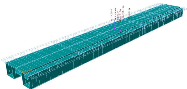
LC-2 하중 재하
